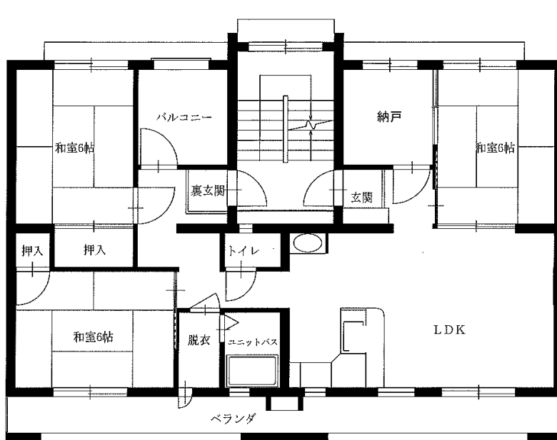
3LDK(6-101・7-301)
