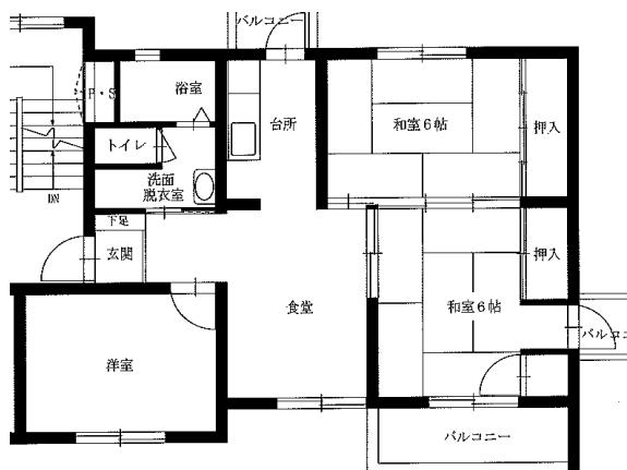
3DK(2-403)
