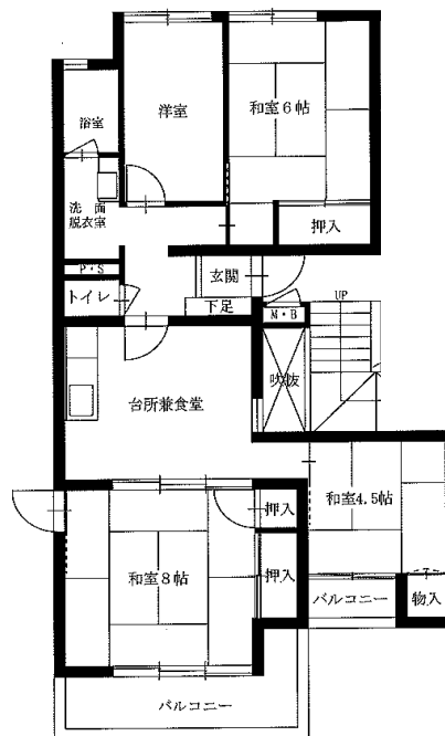
4DK(1-201)
